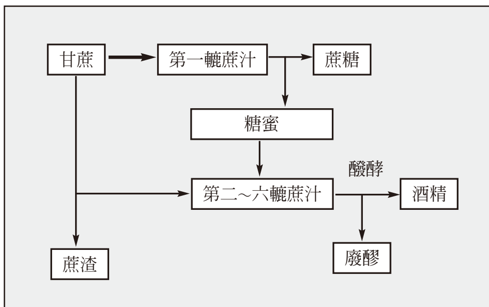
圖一 利用甘蔗同時生產蔗糖、酒精的流程示意圖
