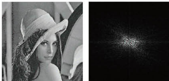
◎左邊的圖經傅立葉轉換後而得的頻譜圖
